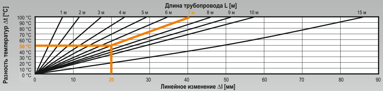
Граф - Линейное изменение трубопровода FIBRE
